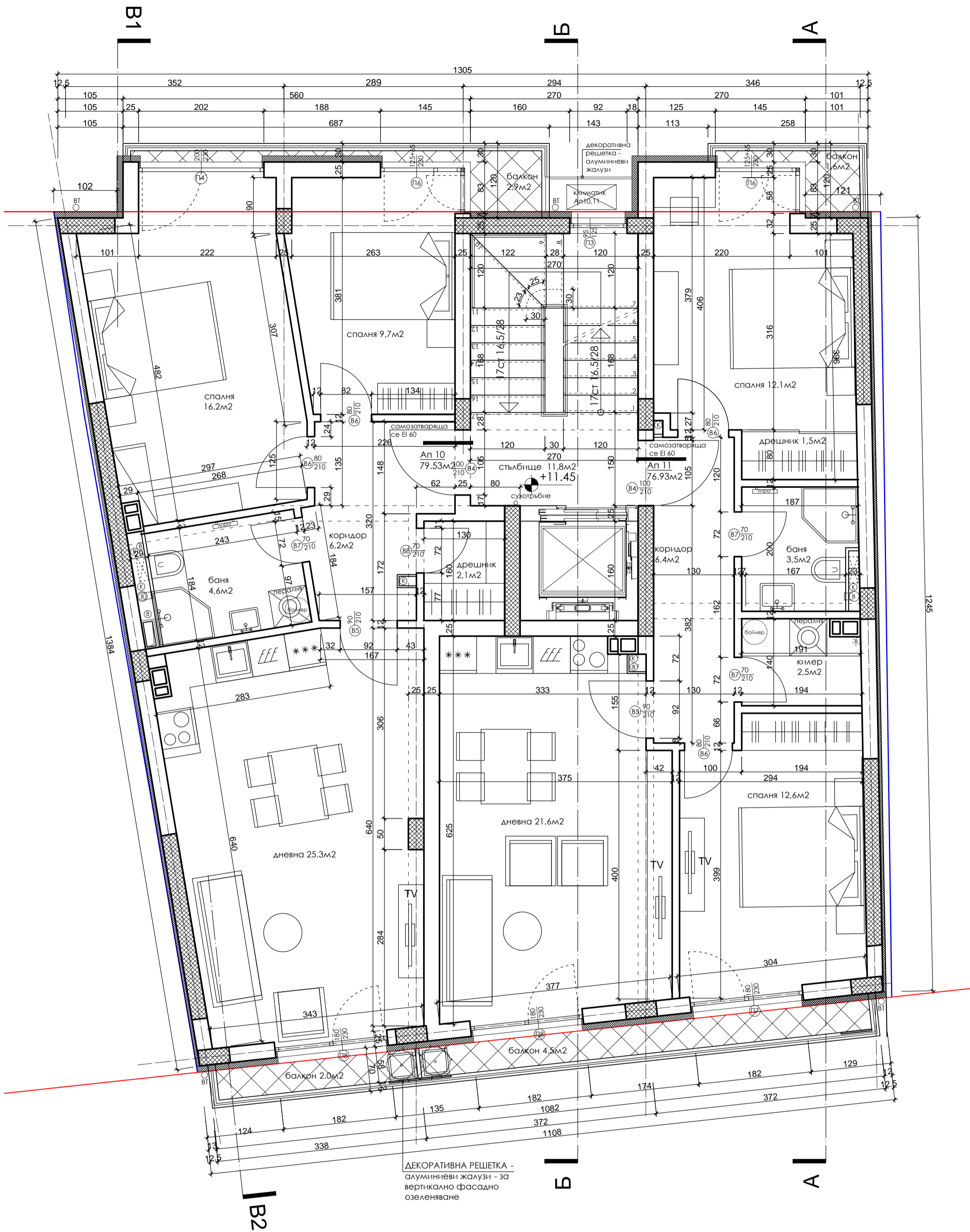
ПЛАН 5 ти ЕТАЖ - 177.7m2
