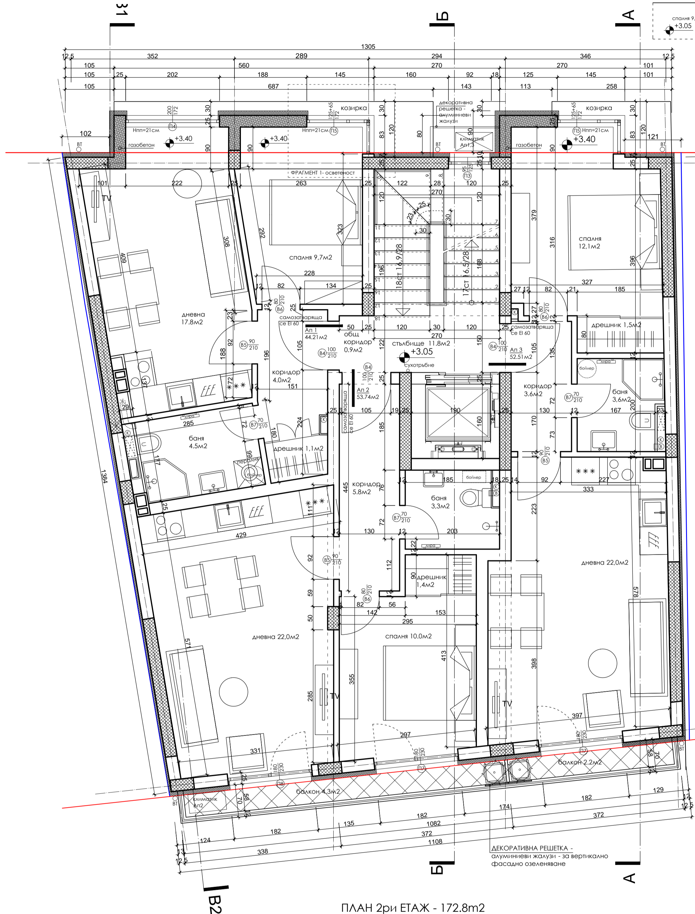
ПЛАН 2ри ЕТАЖ - 172.8м2
